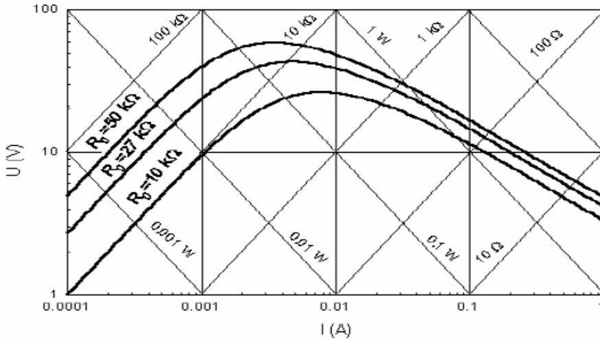
Influența temperaturii ambiante asupra caracteristicii U(I) a termistorului NTC
