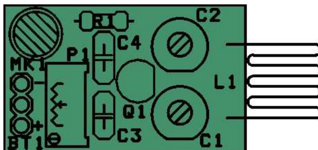
Amplasarea componentelor
