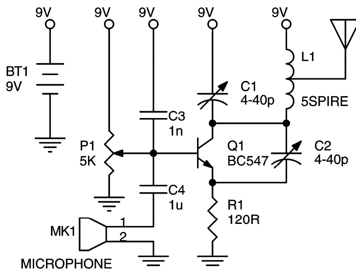
Schema electrică
