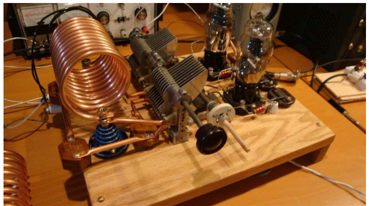
Emițătorul Colpitts
